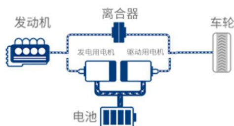
图 23：本田 i-MMD 混动系统构型原理图
