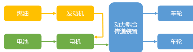
图 7：混动汽车工作模式—串联驱动
