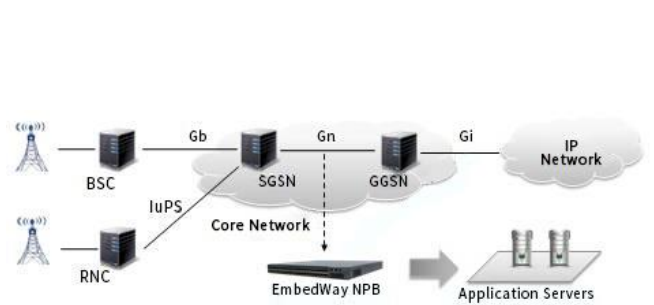
图 12: GSM/WCDMA/TD-SCDMA 核心网采集分流解决方案
