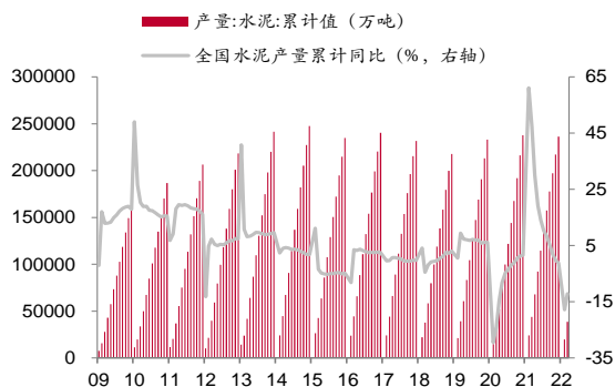
图表 62: 全国水泥产量及同比增速
