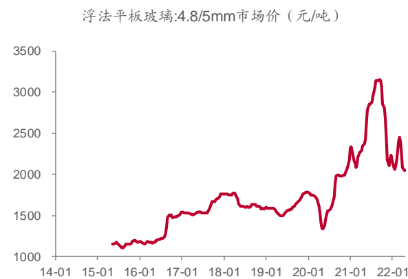
图表 18: 浮法平板玻璃市场价 (元/吨, 4.8/5mm)
