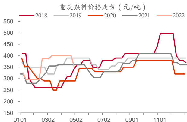
图表 43: 重庆熟料价格 (元/吨)
