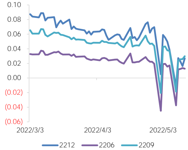
图 2.3.12: 季月合约 (UC-CNH) 基差 (单位: pips)
