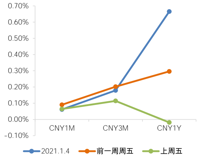
图 2.3.14: 境内外汇掉期曲线 (年化)
