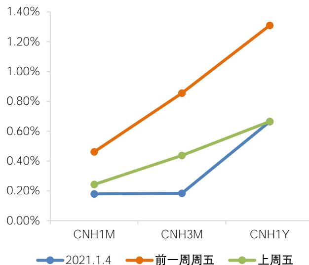
图 2.3.16: 境外外汇掉期曲线 (年化)
