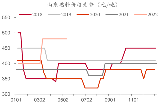
图表 40: 山东熟料价格 (元/吨)
