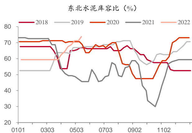
图表 46: 东北水泥库容比 (%)
