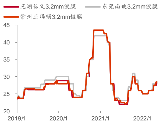
图表 23: 光伏玻璃主要厂商 3.2mm 镀膜价格 (元/平)
