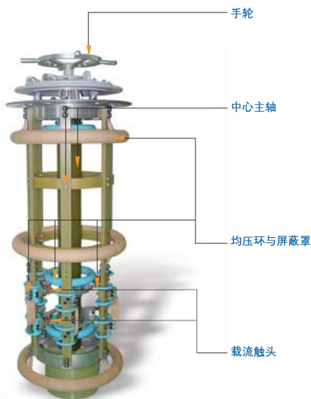
图 14：无励磁分接开关结构图
