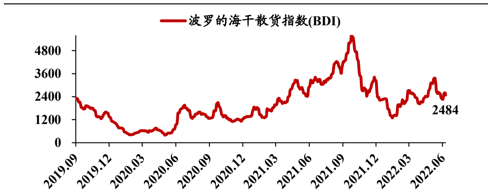
图 25: 6 月 21 日 BDI 干散指数较 6 月 13 日增加 9.9%
