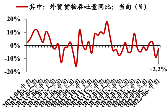
图 2：6 月中旬，沿海主要枢纽港口外贸货物吞吐量同比-2.2%
