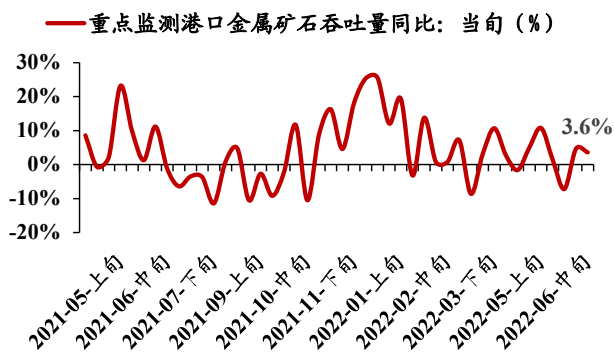
图 9: 6月中旬,重点港口铁矿石吞吐量当旬同比+3.6%
