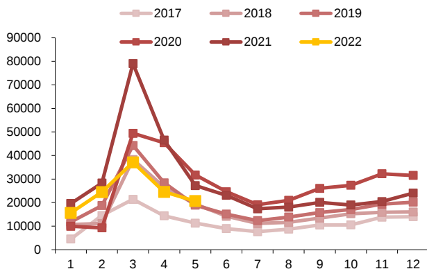
图 18：挖掘机月度销量
