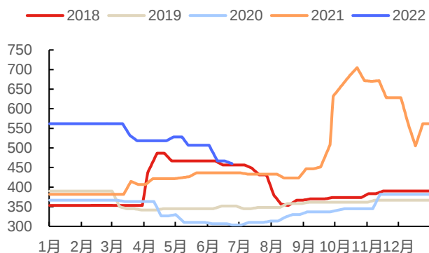
图 23: 2018/1/3-2022/6/17 东北地区水泥均价（元/吨）
