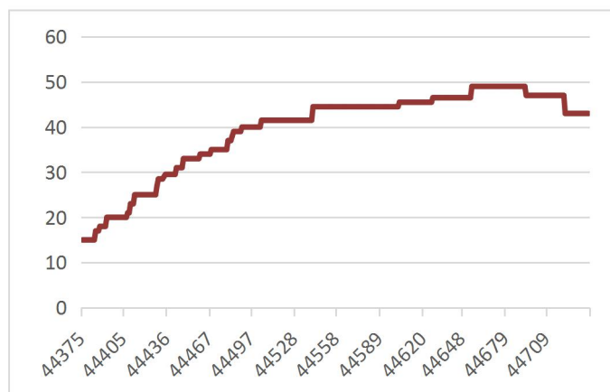
图 13：PVDF（万元/吨）
