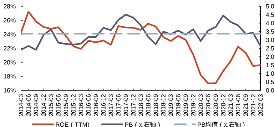
图 38: PB-ROE 视角：一季度 ROE 小幅回升，PB 低于均值
