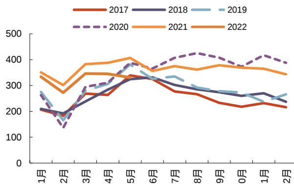
图5：2017年1月-2022年5月冰箱月度出口量（万台）
