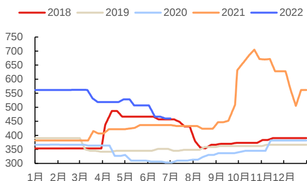
图 23：2018/1/3-2022/7/1 东北地区水泥均价（元/吨）
