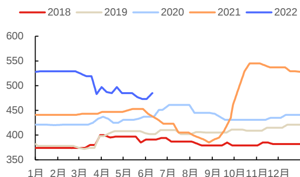
图 24：2018/1/3-2022/7/1 西北地区水泥均价（元/吨）
