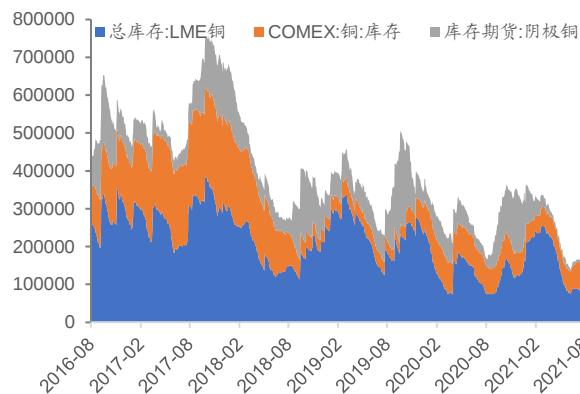
图 14: 铜库存 (吨)
