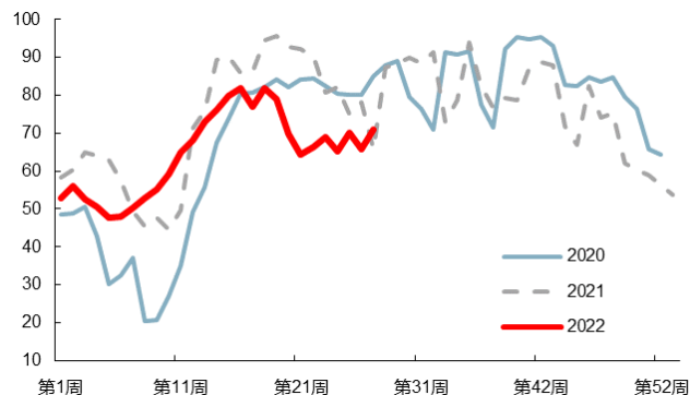
图 30：全国水泥周开工率（%）
