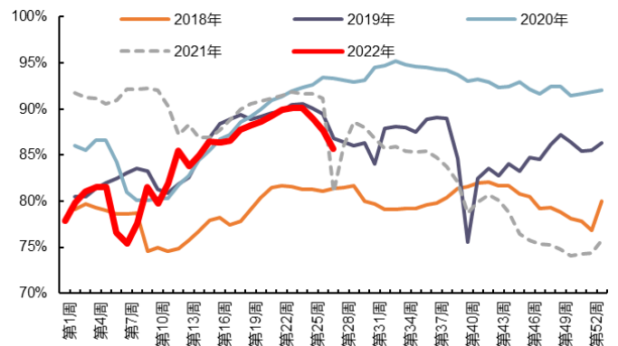
图 26：全国 247 座高炉产能利用率（%）
