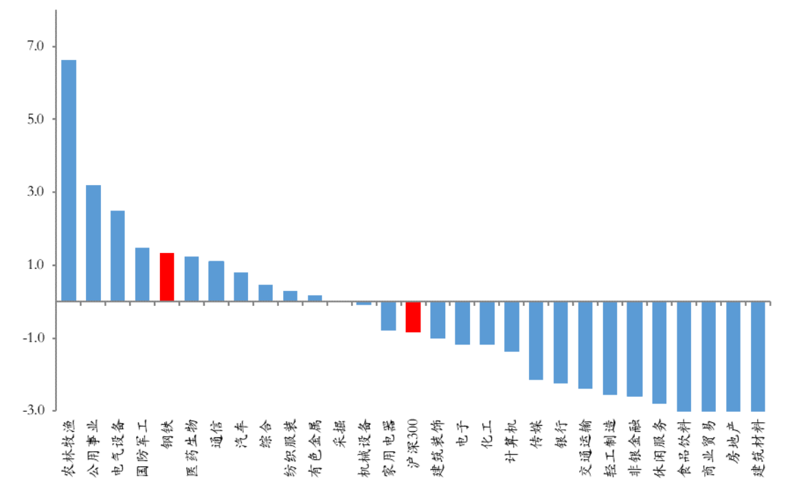
图表 1 本周钢铁板块涨幅为 1.34 百分点 (%)
