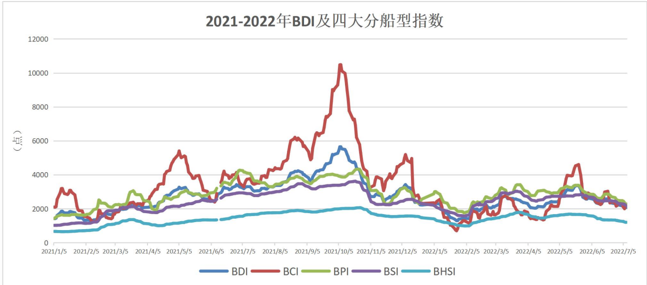
图 2-1：BDI 及分船型指数
