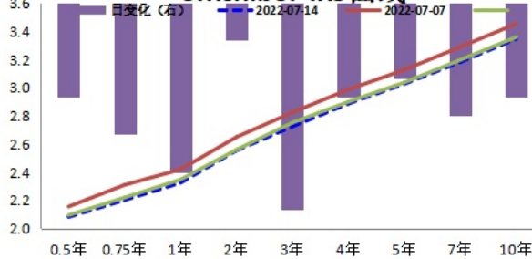
3Mshibor-IRS曲线
