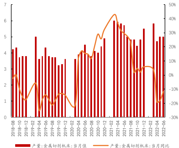
图 17 金属成形机床当月产量及增速（左轴为产量当月值，台；右轴为当月同比，%）
