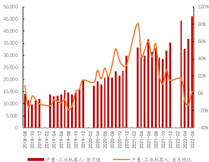
图 11 工业机器人当月产量及增速（左轴为产量当月值，台；右轴为当月同比，%）
