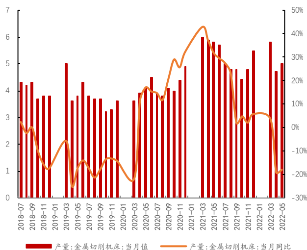
图 15 金属切削机床当月产量及增速（左轴为产量当月值，万台；右轴为当月同比，%）
