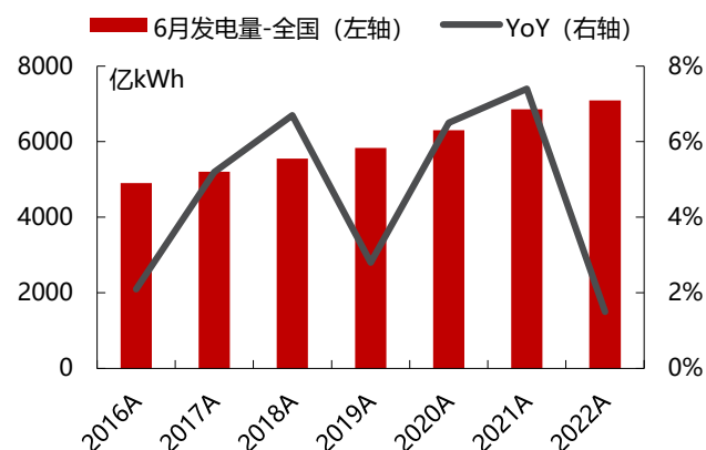
图8：2022年6月全国发电量同比增长1.5%
