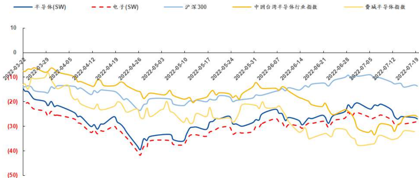
图4: 全球主要半导体指数走势 (%) (截止07/19)
