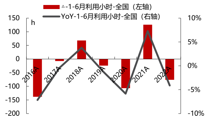
图6：2022年1-6月全国利用小时同比下降4.1%
