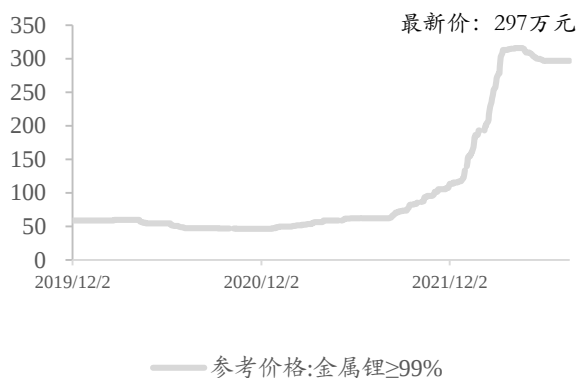
图3：锂价格走势（截至 2022/07/22）
