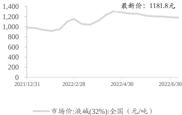
图11: 液碱价格走势 (截至 2022/07/10)
