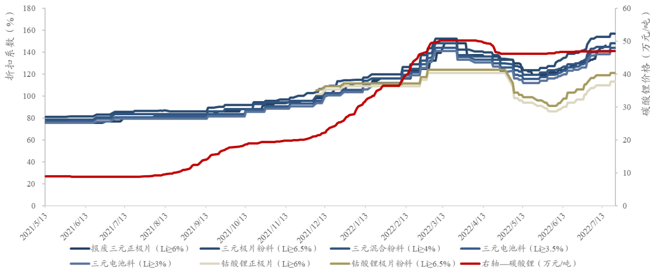
图2：废电池采购折扣系数与碳酸锂价格（截至 2022/07/22）
