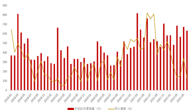
图 18: 推土机月度销量
