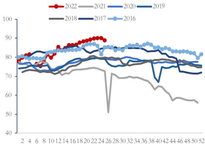
图表 27 全国钢厂高炉产能利用率 (%)
