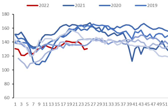
图表 33 全国建材钢厂线材实际周产量（万吨）
