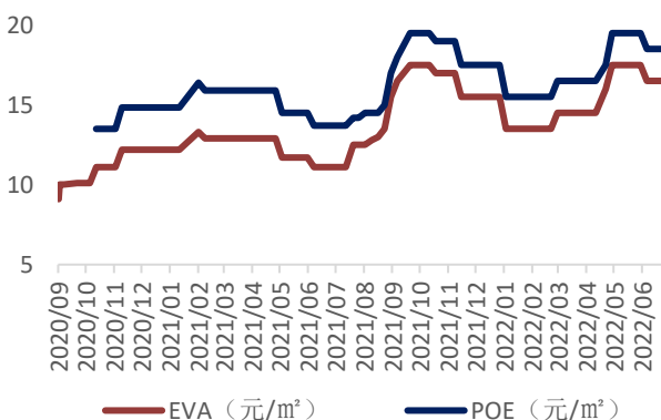
图表 6：EVA 及 POE 分别 16.5 元/㎡、18.5 元/㎡
