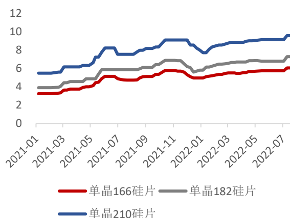
图表 2：单晶 182 硅片 7.28 元/W，环比 0%（20220724）
