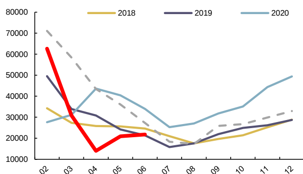
图 33：挖掘机产量（台）
