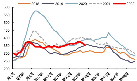
图 22：热轧板卷周度库存（万吨）
