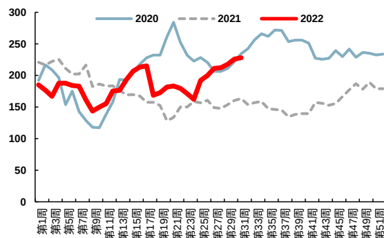
图 74: 110 家样本洗煤厂精煤库存 (万吨)
