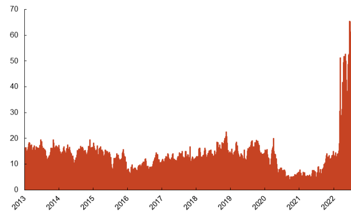
图 45：新加坡柴油-原油价差（美元/桶）
