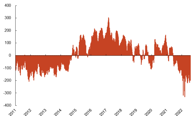
图 42：PDH 价差（美元/吨）
