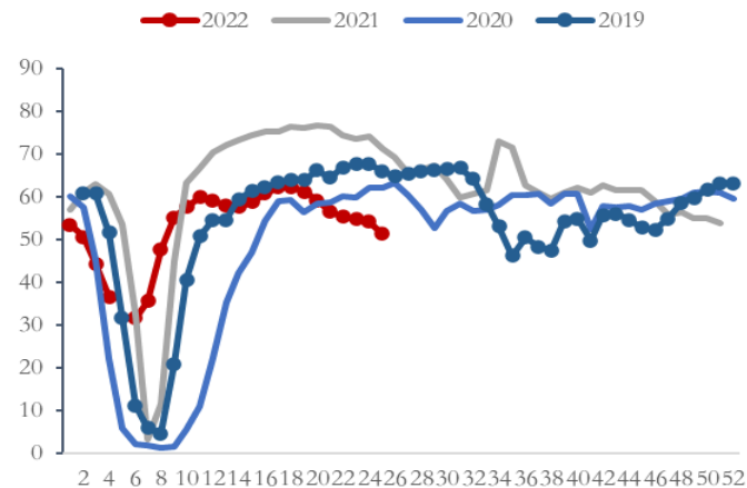
图表 29 样本钢厂电炉产能利用率: 全国 (%)
