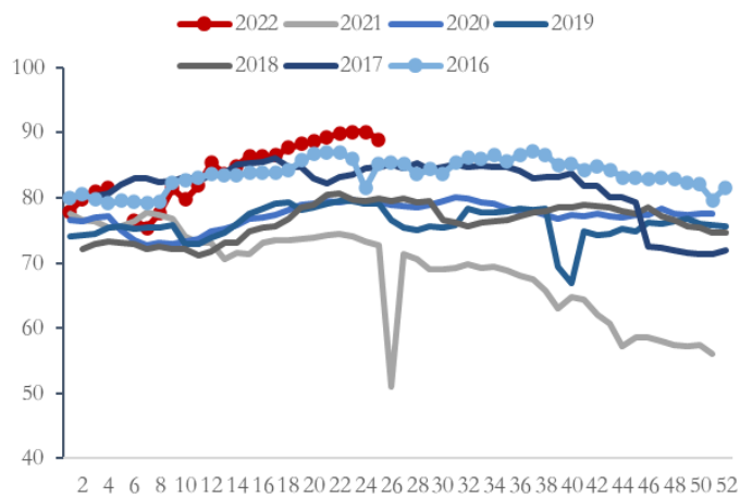
图表 27 全国钢厂高炉产能利用率 (%)
