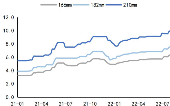
图2: 硅片价格走势 (元/片)
