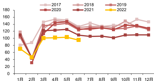
图 13：小松中国挖掘机利用小时数（小时）
