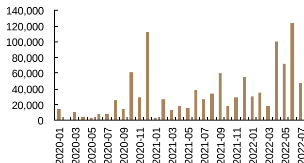
图 5：我国充电桩月度新增数（台）
