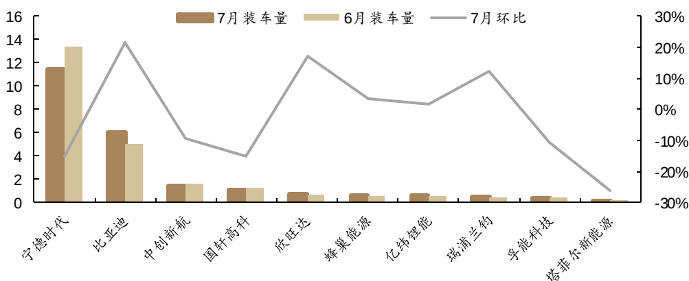
图 11：我国7月国内动力电池企业装车量前十名装车量（GWh）及环比
