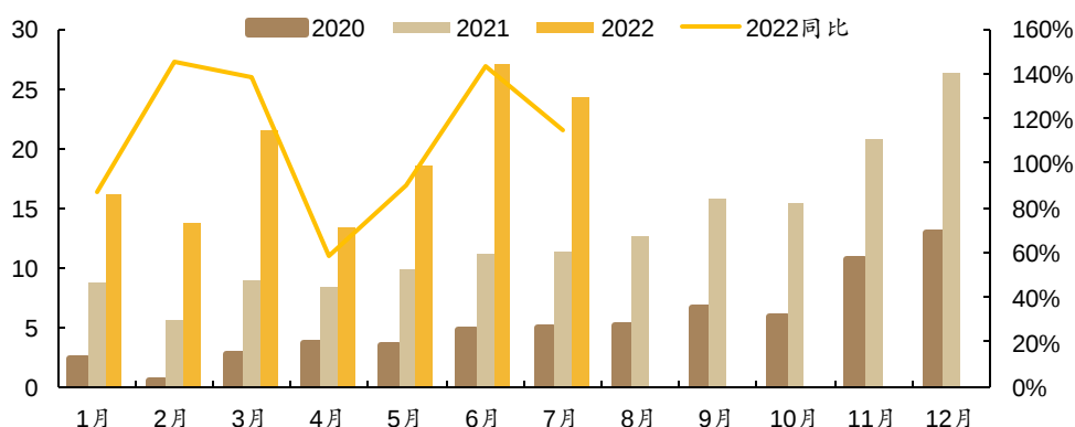
图 9：我国 2020 年 1 月-2022 年 7 月电池装机量情况（单位：GWh）
