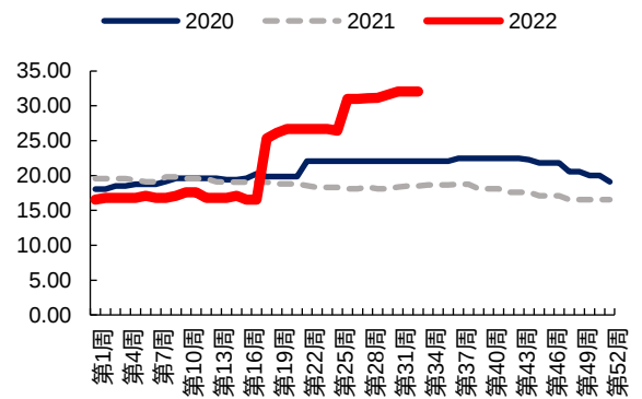
图 60：光伏玻璃周度产量(万吨)
