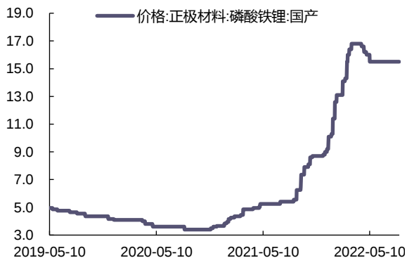
图 27: 磷酸铁锂价格(万元/吨)
