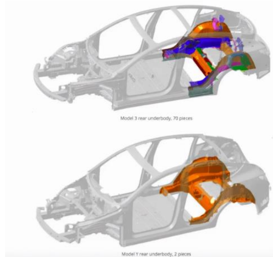
图17：特斯拉后底板零件数量减少
