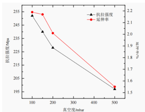
图22: 不同真空度下产品力学性能的对比
