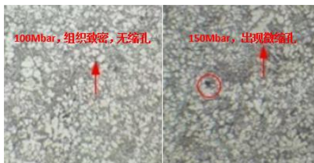
图23: 100mbar 和 150mbar 下压铸产品金相对比
