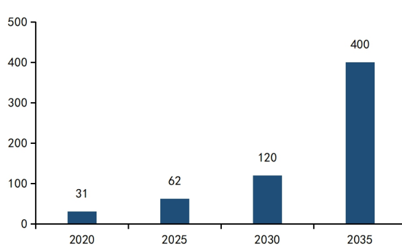
图16: 我国中长期抽水蓄能发展规划装机容量 (GW)
