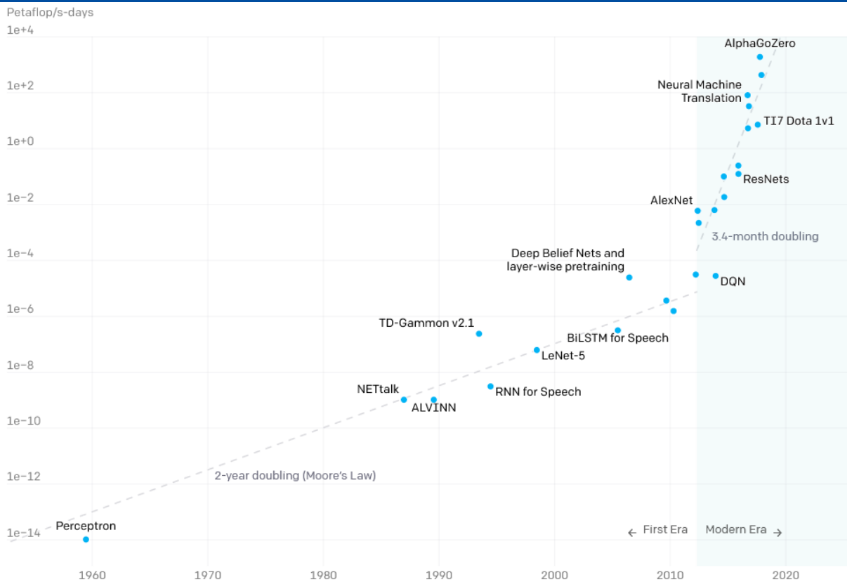
图 36. 主要人工智能模型算力需求一览（1960-2020 年）
