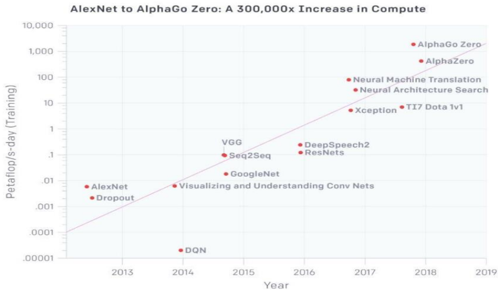
图 18. AI 算力需求剧增 30 万倍（2013-2019）
