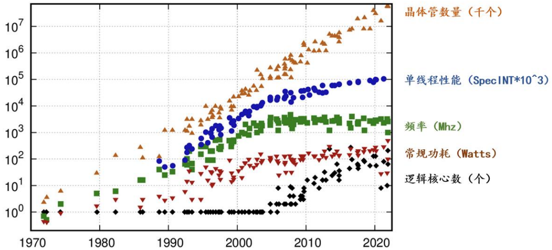
图 37. 过去五十年微处理机芯片趋势数据（1970-2020 年）
