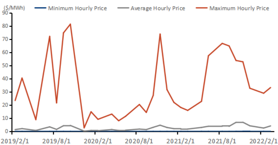
图：2019年2月-2022年3月PJM市场峰谷价差
