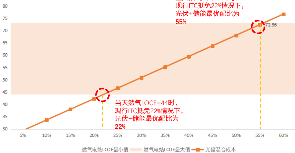
图：现行ITC（22%）-不同储能功率配比的4H光储电站加权LCOE与天然气机组对比($/MWh)
