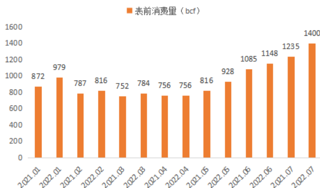
图：天然气表前端消费量
