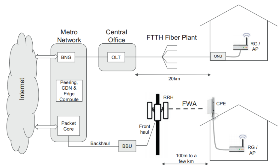
图2：FTTH 和 FWA 传输路径
