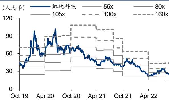
图表3: 虹软科技 PE-Bands
