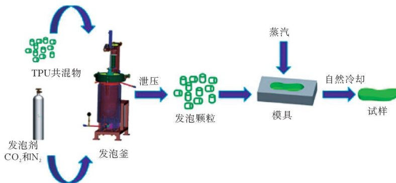
图表 19 TPU 发泡鞋材工艺过程
