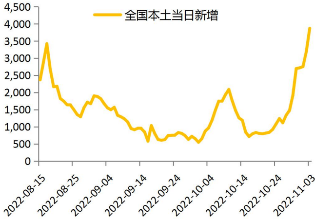
图 14: 全国当日新增确诊 (例)
