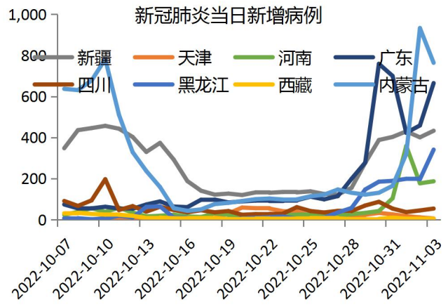
图 15: 主要城市当日新增确诊+无症状 (例)
