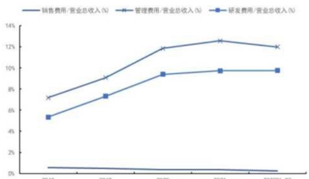
图6: 国博电子三项费用率 (单位: %)
