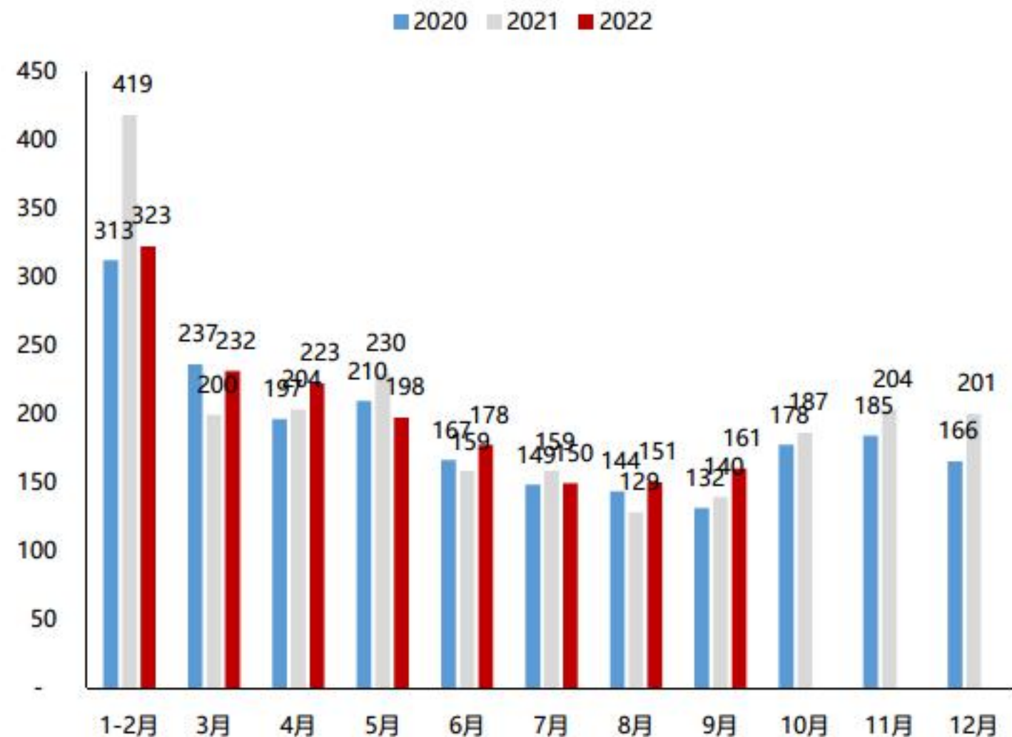
图：全国风电项目平均利用小时数
