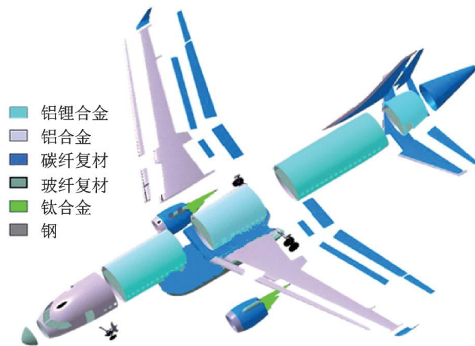
图30 C919 全机材料使用图
