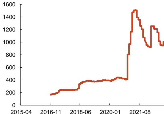
图 90：99.95%铀价格(元/克)
