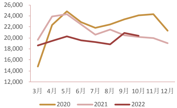
图 6：全国水泥（月度）产量（吨）
