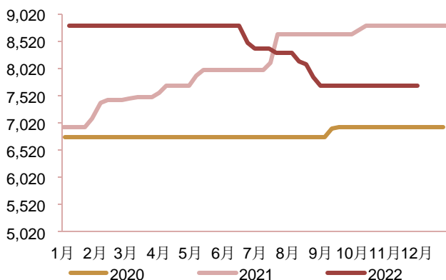
图 42：短切纱均价（元/吨）
