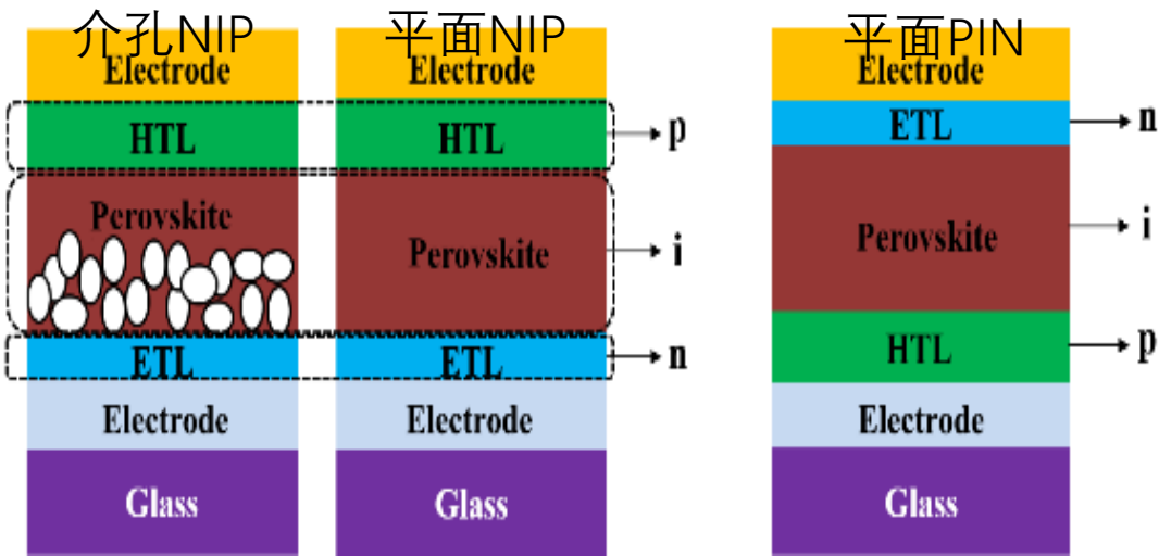
图表：钙钛矿电池基本结构
