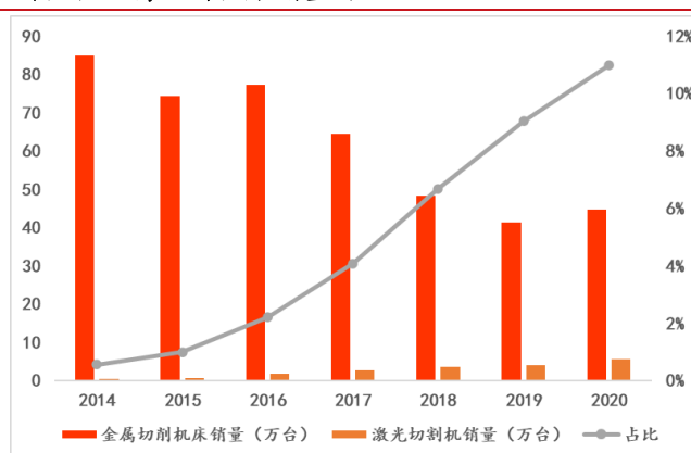
图表46：中国激光切割机和金属切削机床销量对比
