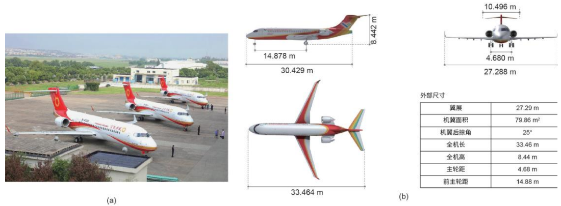
图31 ARJ21 新支线飞机
