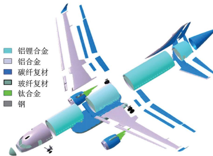
图35 C919 全机材料使用图
