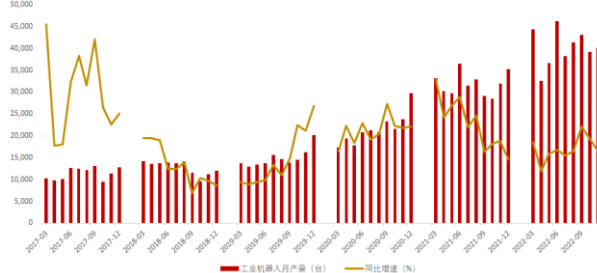
图 27：工业机器人月度产量及增速（台，%）
