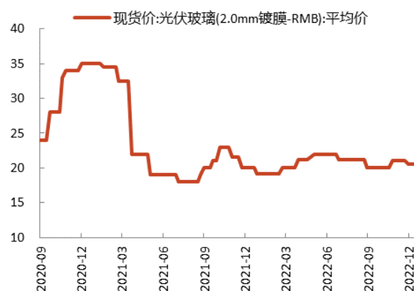
图 14：2mm 光伏玻璃价格（元/平米）
